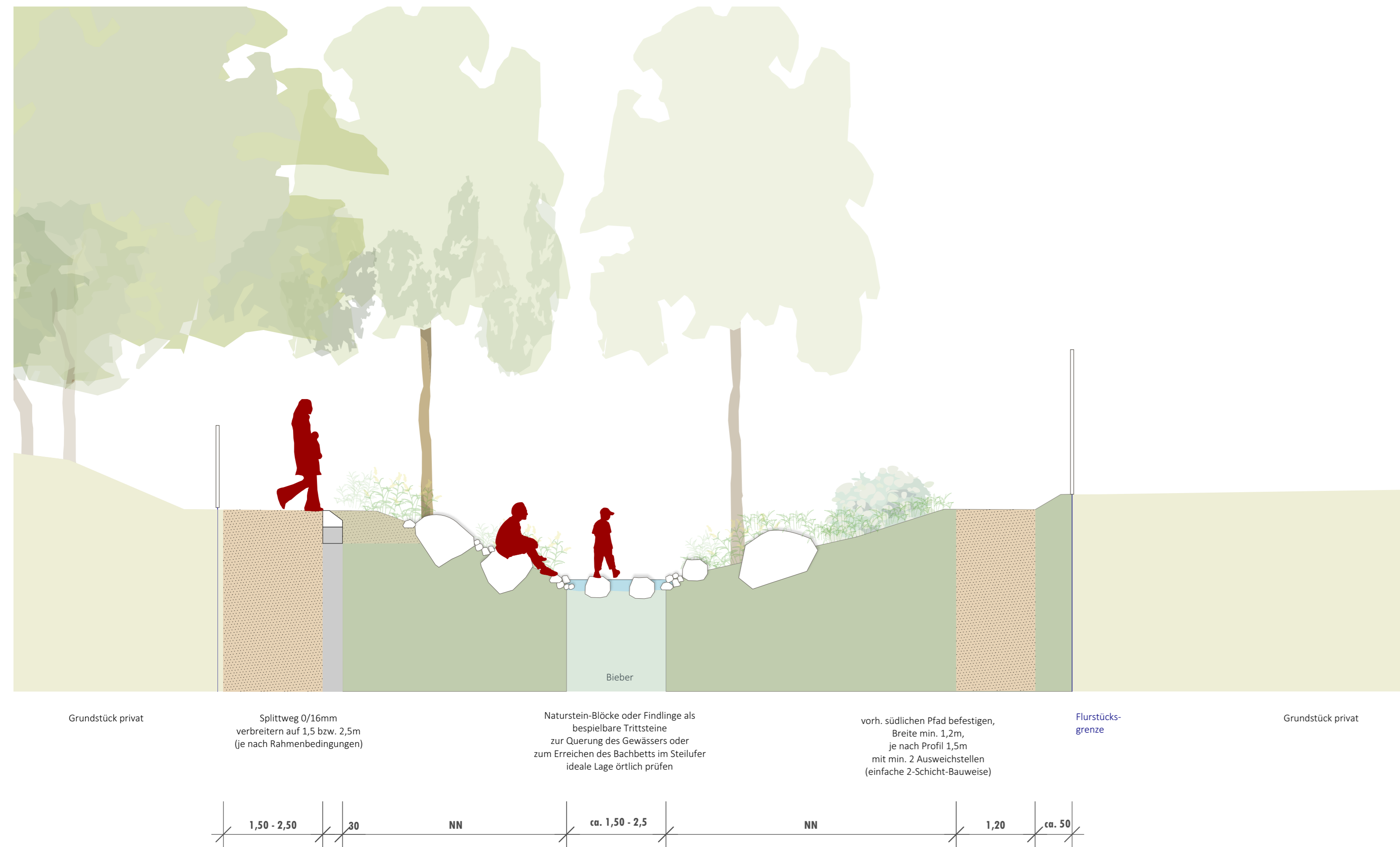
Schemaschnitt Ost M 1:50 Bieberpromenade + Bieberpfad rechts und links des Gewässers
